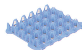
エッグトレイ 20-2A 外寸:315×235×49
