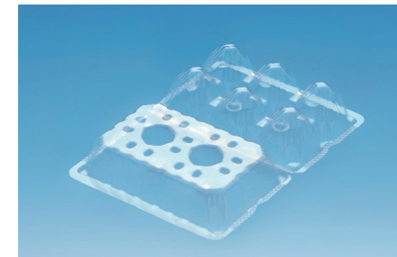
6H 平面 (テープシール) 寸法 (mm) : 150×211×39 ケース入数 (枚) : 2,400
