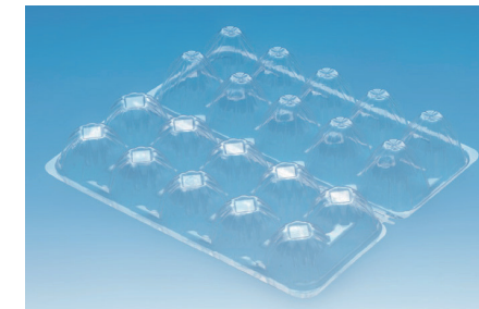
Cパック 10H 寸法 (mm) : 255×225×42 ケース入数 (枚) : 1,200
