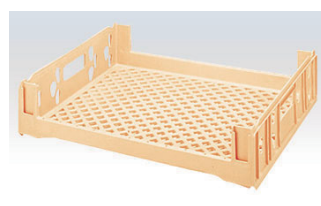
E-24 外寸：652×532×151
