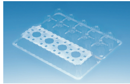
10H 平面 寸法 (mm) : 243×213×39 ケース入数 (枚) : 1,600
