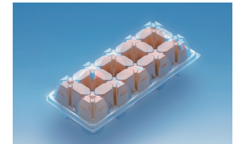
KanKanパック (10H平面カンゴウ式) 寸法 (mm) : 247×220×38 ケース入数 (枚) : 900
