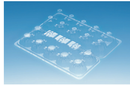
10H 内側面3連結 寸法 (mm) : 245×220×39 ケース入数 (枚) : 1,600
