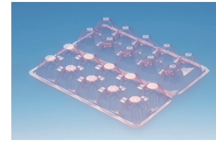
10HLL 赤 寸法 (mm) : 252×222×39 ケース入数 (枚) : 1,600
