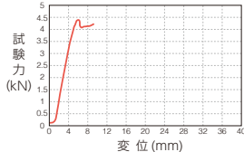
天板曲げ強度：4.5kN
