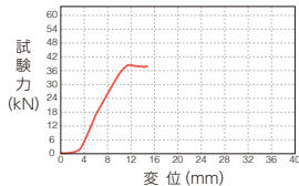
全面圧縮強度：38.0kN
