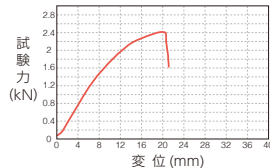
パレット曲げ強度：2.4kN
